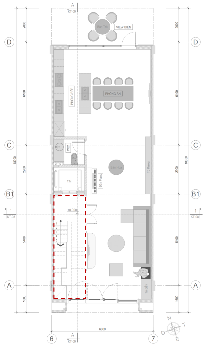
MẶT BẰNG HOÀN THIỆN TẦNG 1
