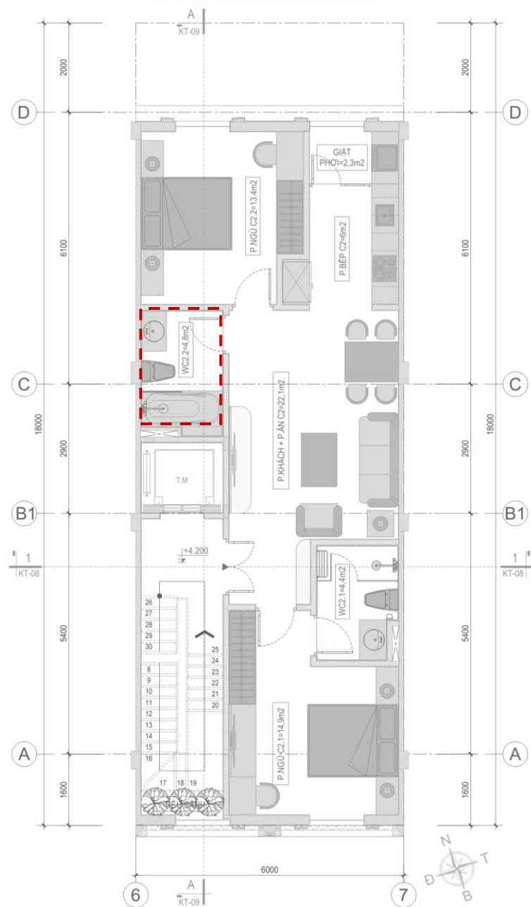
MẶT BẰNG HOÀN THIỆN TẦNG 2
