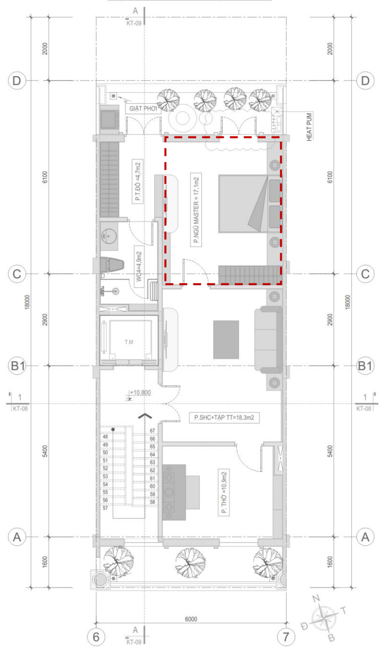
MẶT BẰNG HOÀN THIỆN TẦNG 4
